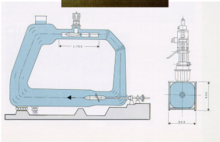
Túnel de Cavitación
