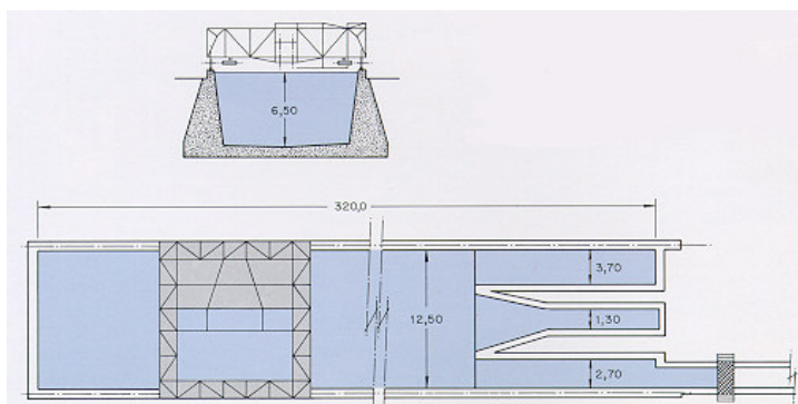
Canal de Aguas Tranquilas
